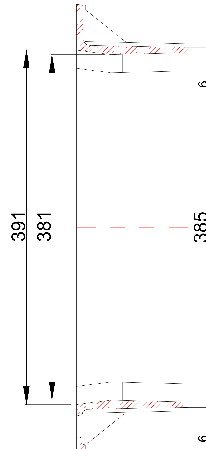
SECTION 0N D-D SCALE 1:2
