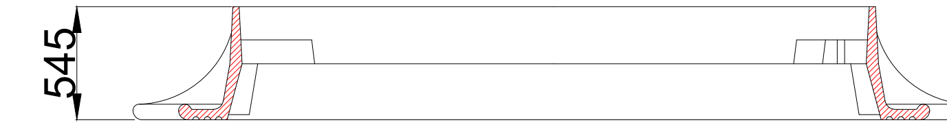
SECTION A-A
